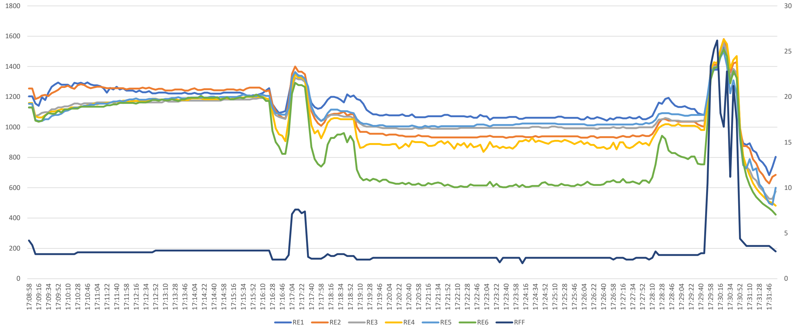
Right Engine EGT & FF
