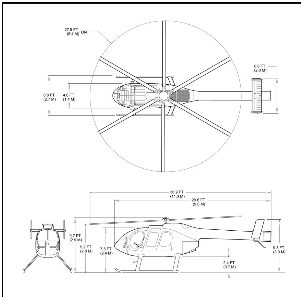
MD 600N External Dimensions
